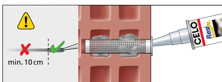
4. Vyhodte prvních 10 cm. Vytlačte potřebné množství chemické kotvy (zcela zaplňte kotvení sítko)
