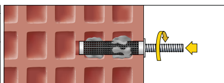
5. Šroubovým pohybem zatlačte kotvení tyč
