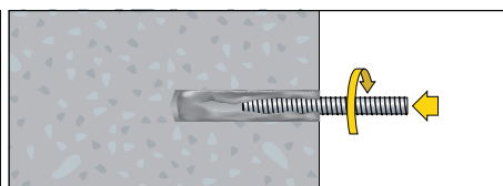
4. Šroubovým pohybem zatlačte kotvení tyč
