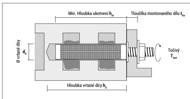
5. Šroubovým pohybem zatlačte kotvení tyč
