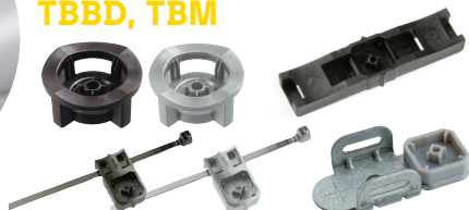
Kabelové přichytky s vázacími pásky TBB, TBBL, TBBD, TBM
